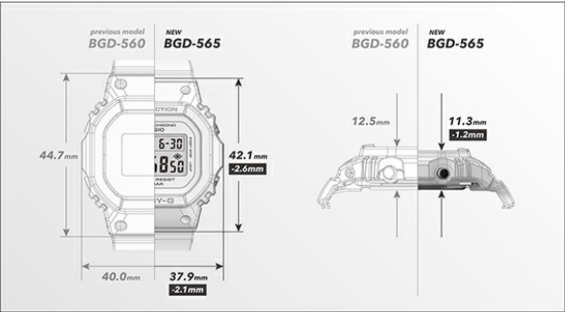
BGD-560とBGD-565のサイズ比較
