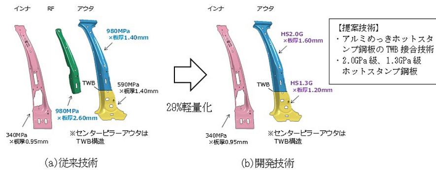
図6 2.0GPaホットスタンプTWB構造によるセンターピラー軽量化技術
