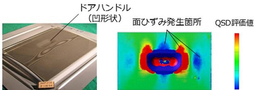
図9 NSa®-QSDによる面ひずみ発生領域の可視化
