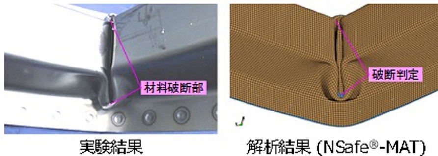
図7 NSa®-MATによる材料破断予測
