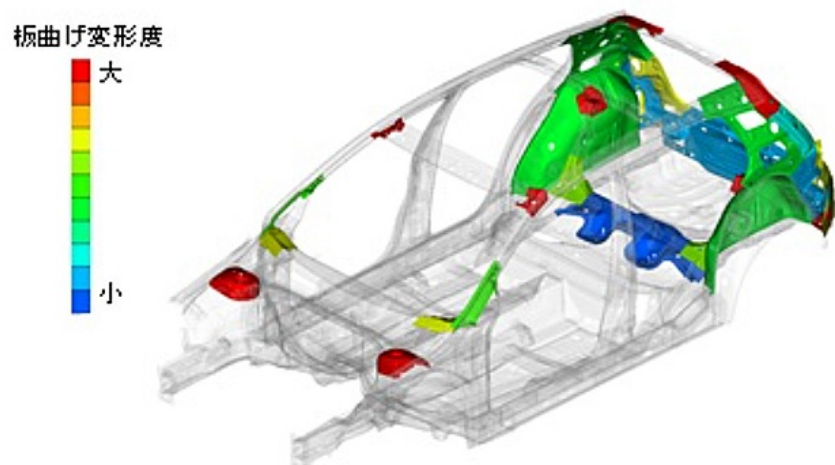
図 10 NS ® -SVを用いた剛性可視化
