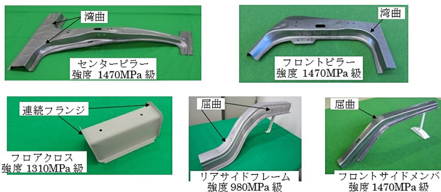
図4 開発工法による超高強度鋼板部品
