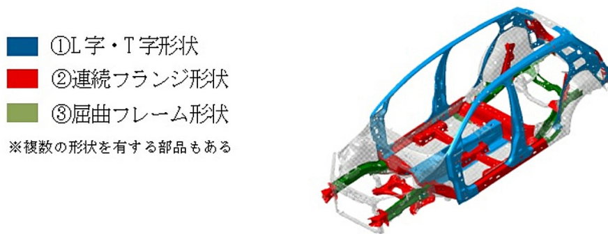
図2 開発工法の適用対象部品
