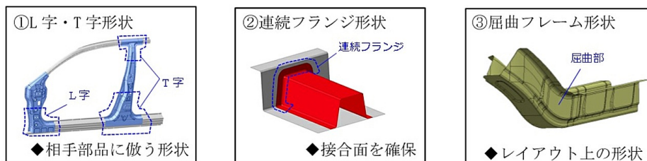
図3 成形困難な結合部形状
