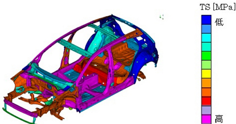
図1 NSafe® -AutoConceptで想定する車体向け鋼材の強度
