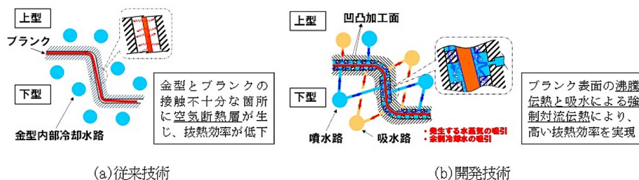
図5 直水冷高生産ホットスタンプ技術
