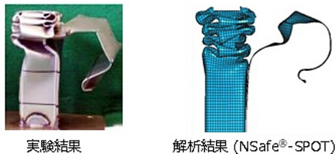
図8 NSa®-SPOTによるスポット溶接部破断予測
