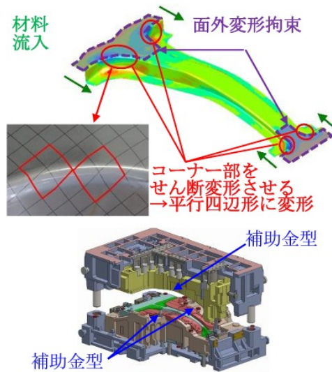
図2. 開発工法専用金型
