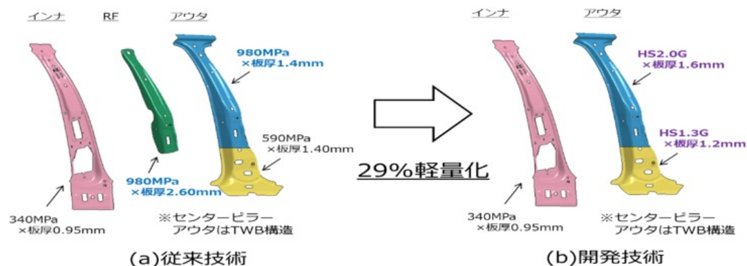
図1 AL-HS鋼板を用いたTWB技術の活用事例
