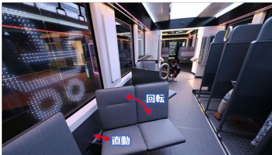
クロスシート配列から、ロングシート配列への変換 [導入製品] LMガイド (HSR)、回転ベアリング (MPG)
