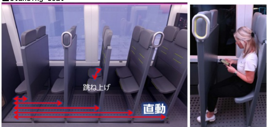
立ち乗りシートのピッチ変換、混雑時に車内空間創出 [導入製品] LMガイド (HSR)
