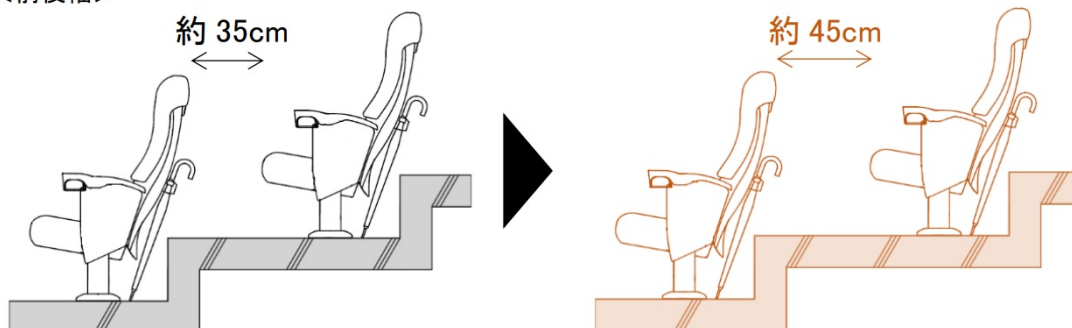
<前後幅>
