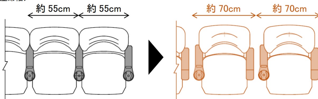
<座席幅>
